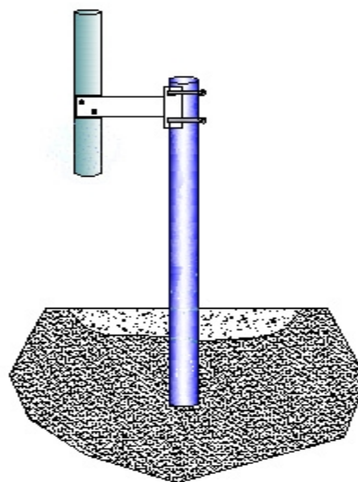
Установка извещателя «Радий-6» в грунт
