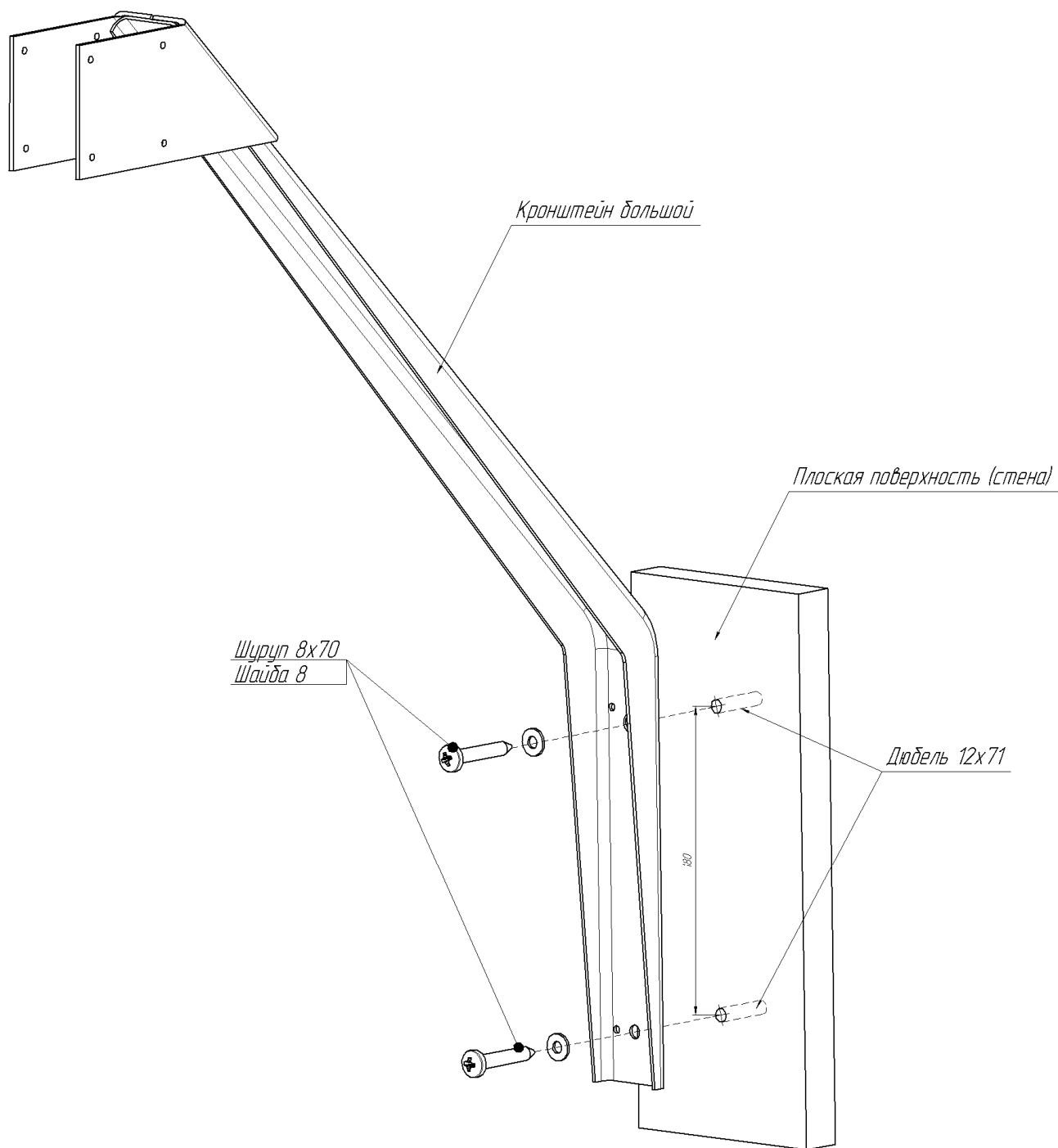
Рисунок 2 – Крепление КМЧ на плоской поверхности
