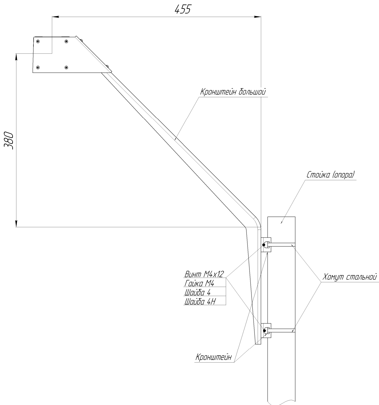
Рисунок 1 – Крепление КМЧ на стойке
