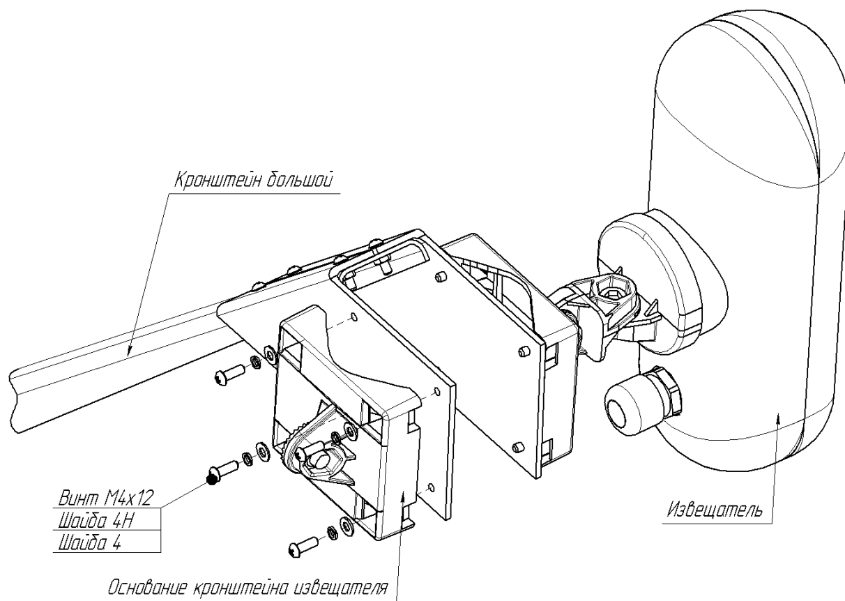
Рисунок 3 – Крепление блока извещателя к КМЧ
