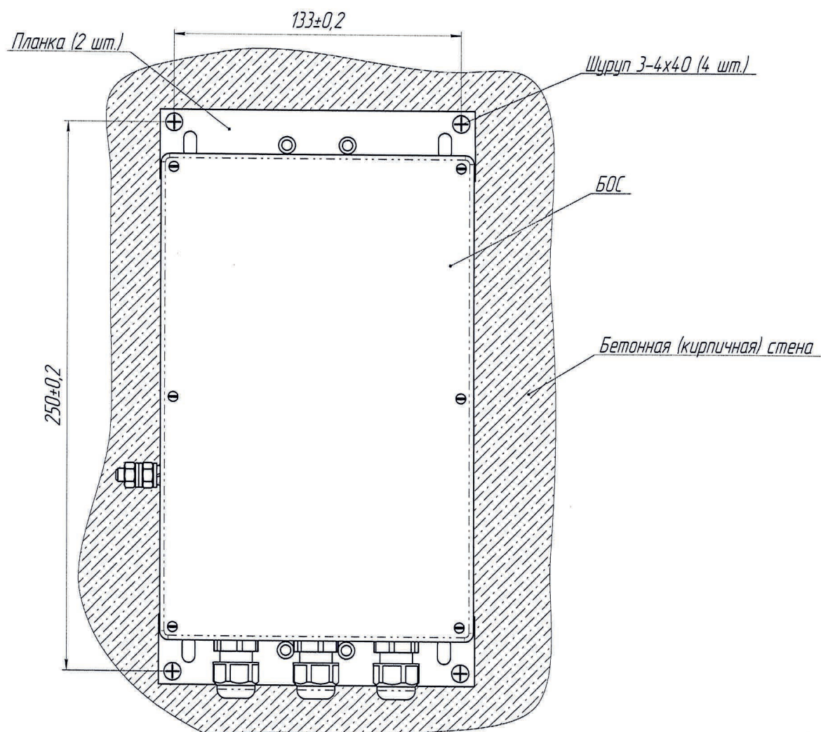
Рисунок 2.3 – Установка БОС на бетонном ограждении
