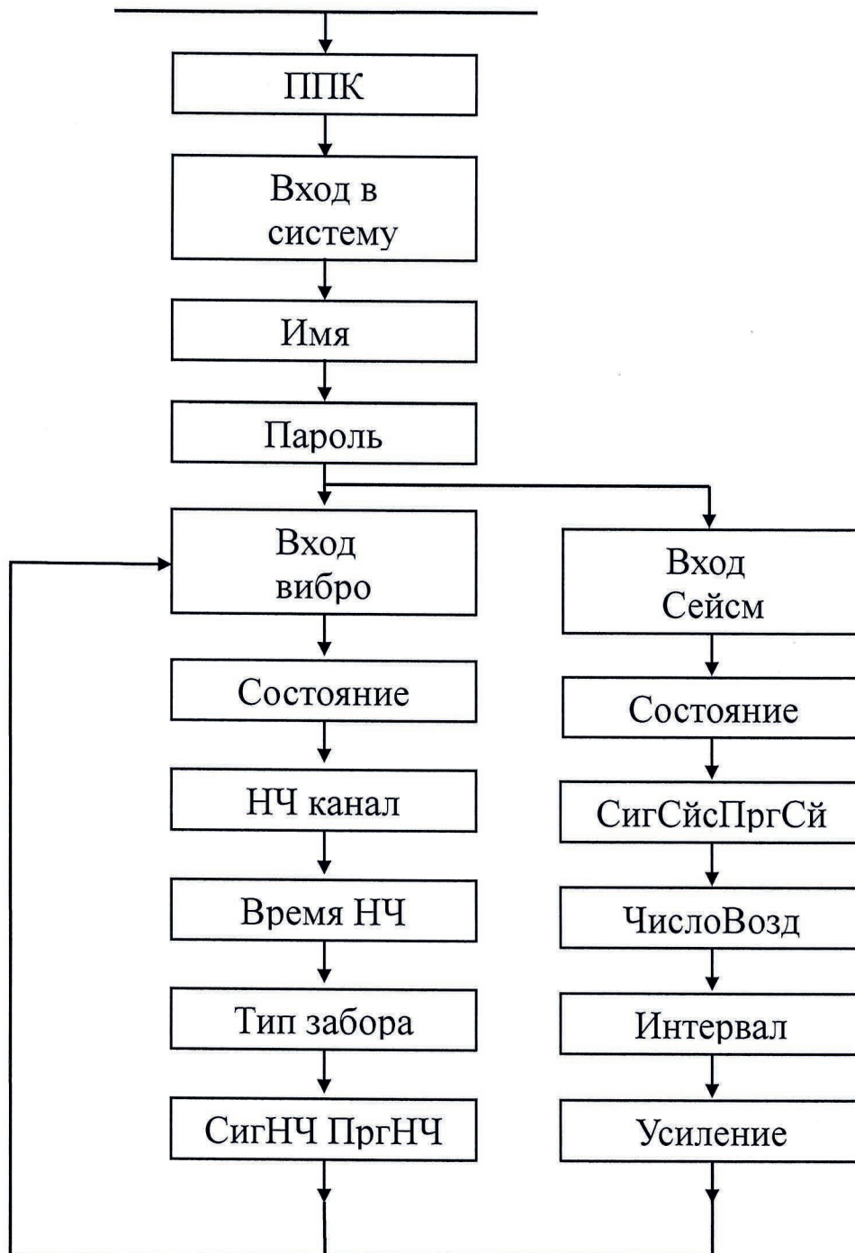
Рисунок Б.2 - Структура меню ППК
