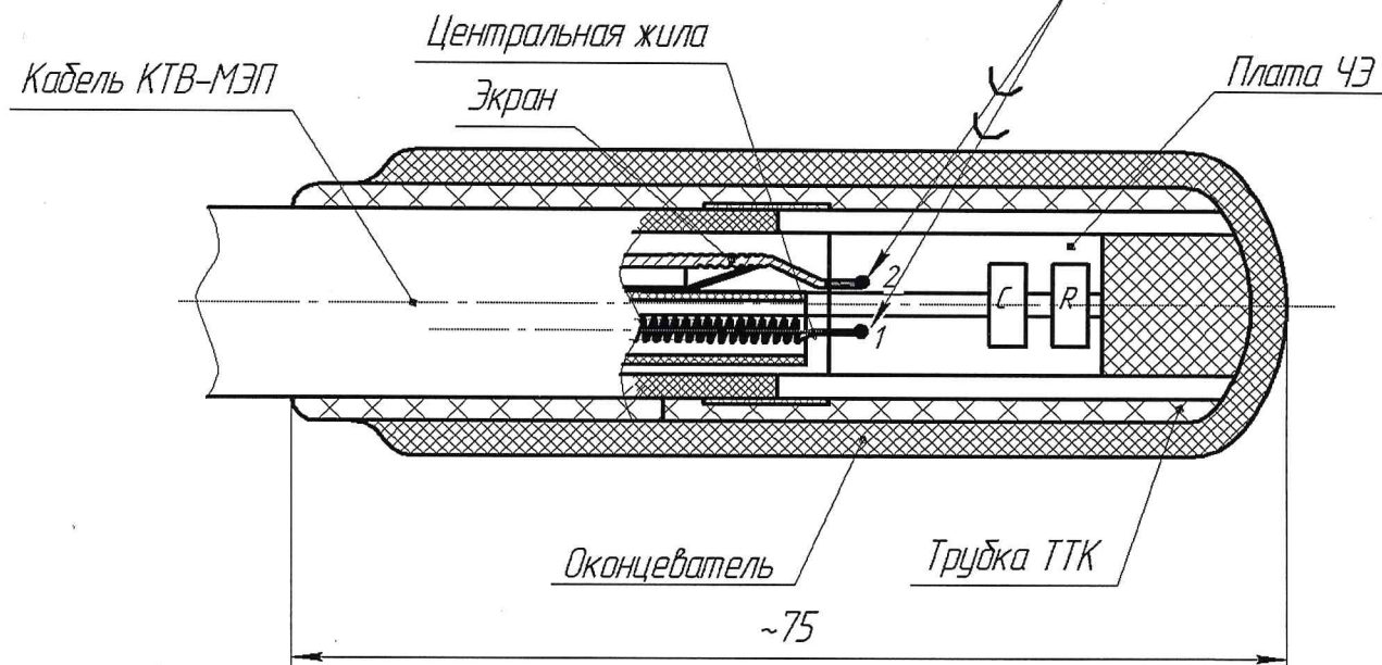
Рисунок 1 – Монтаж ОУ на кабеле СЧЭ КТВ-МЭП
