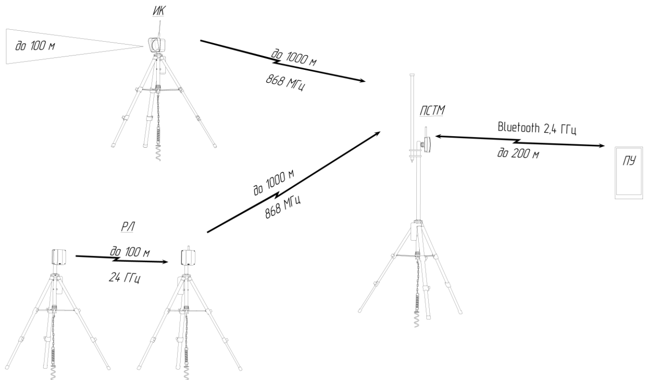
Рисунок 1.4 – Схема взаимодействия составных частей комплекса без RTP (комплект приемника на базе ПСТМ+ПУ)
