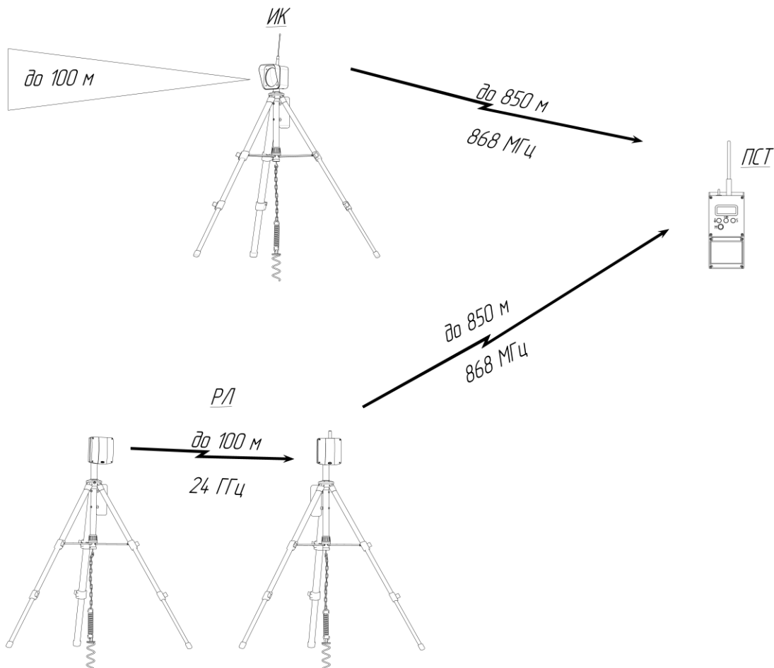
Рисунок 1.3 – Схема взаимодействия составных частей комплекса без RTP (комплект приемника на базе ПСТ)
