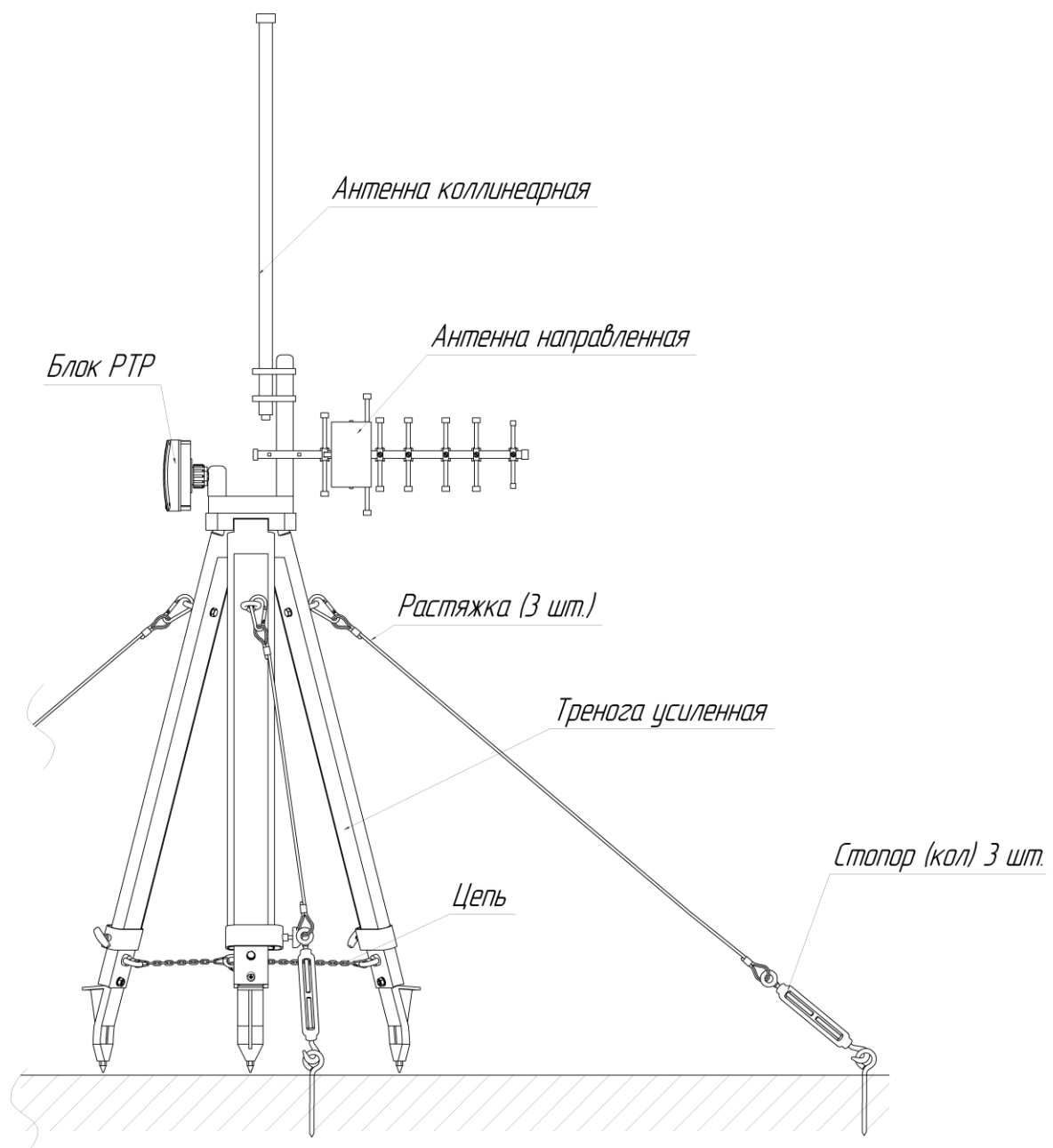
Рисунок 1.19 – Внешний вид РТР, установленного на треноге
