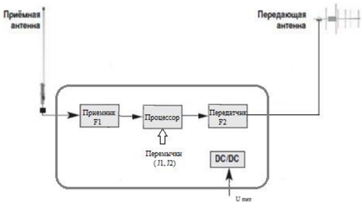
Рисунок 1.17 – Схема функциональная РТР
