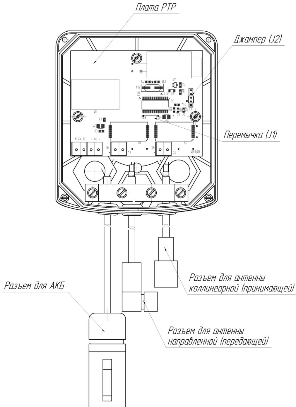
Рисунок 1.18 – РТР со снятой крышкой
