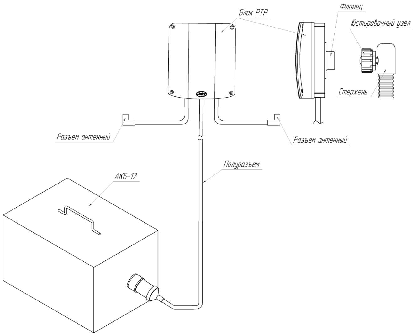
Рисунок 1.20 – Основные элементы РТР
