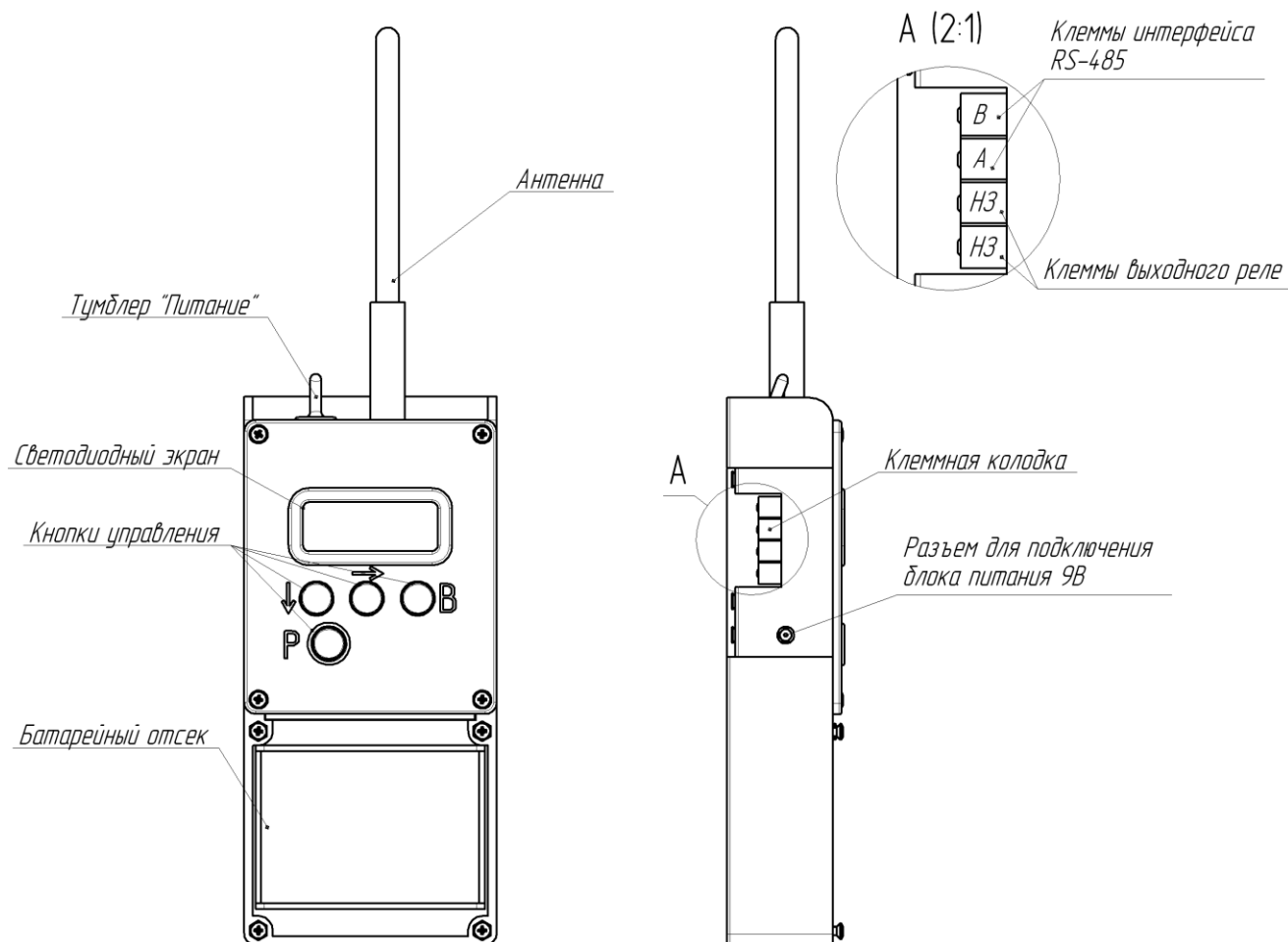
Рисунок 1.13 – Внешний вид блока ПСТ
