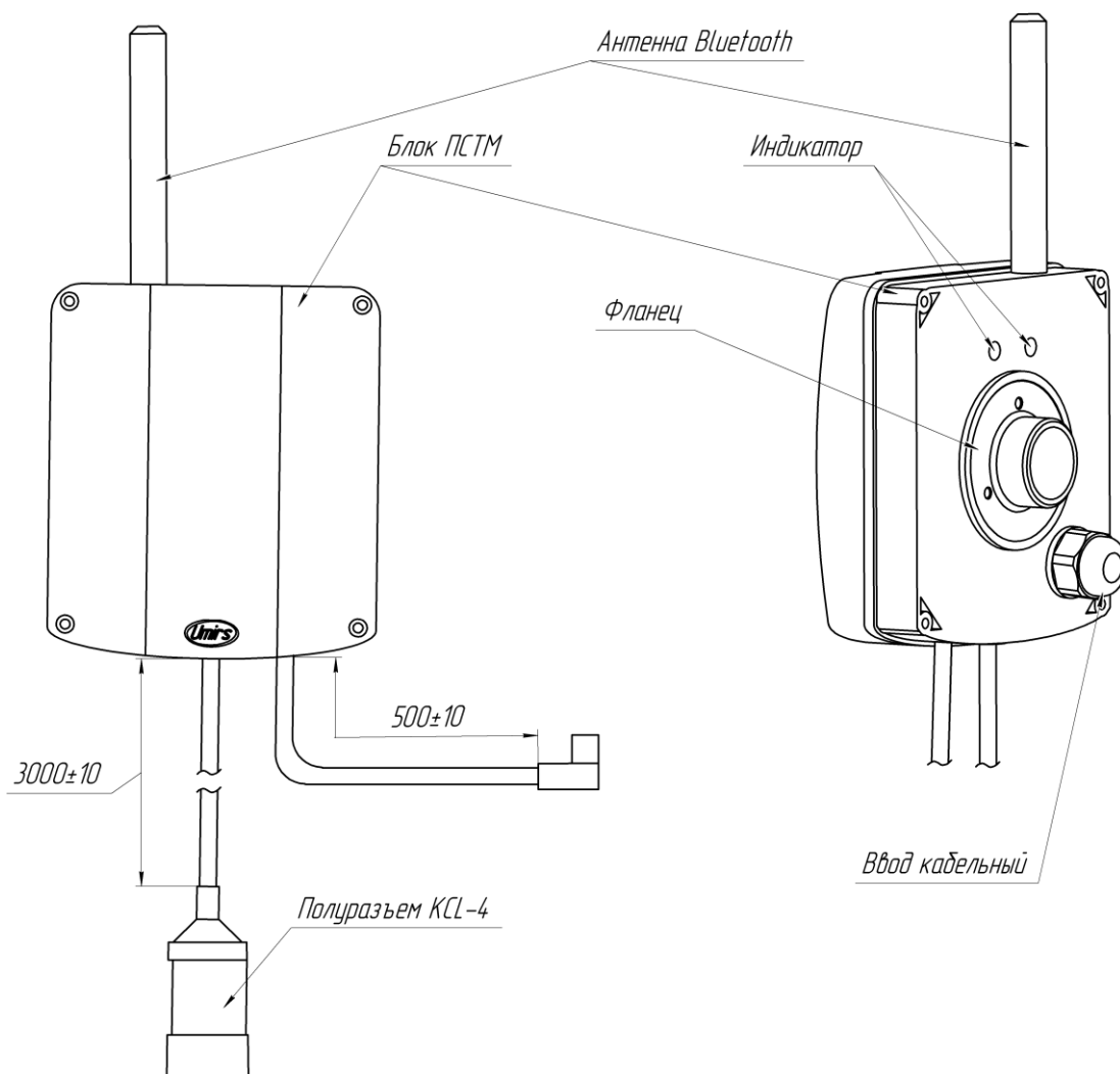
Рисунок 1.14 – Внешний вид блока ПСТМ
