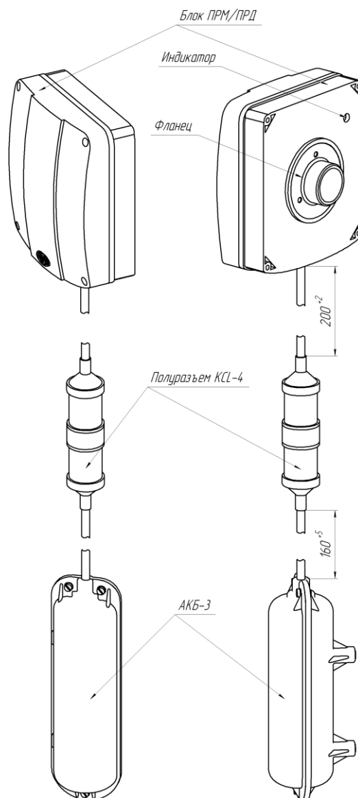
Рисунок 1.7 – Внешний вид ПРМ/ПРД с АК
