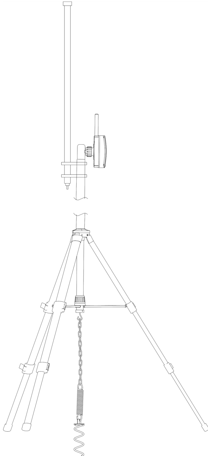
Рисунок 1.15 – Внешний вид ПСТМ на стойке (растяжки не показаны)
