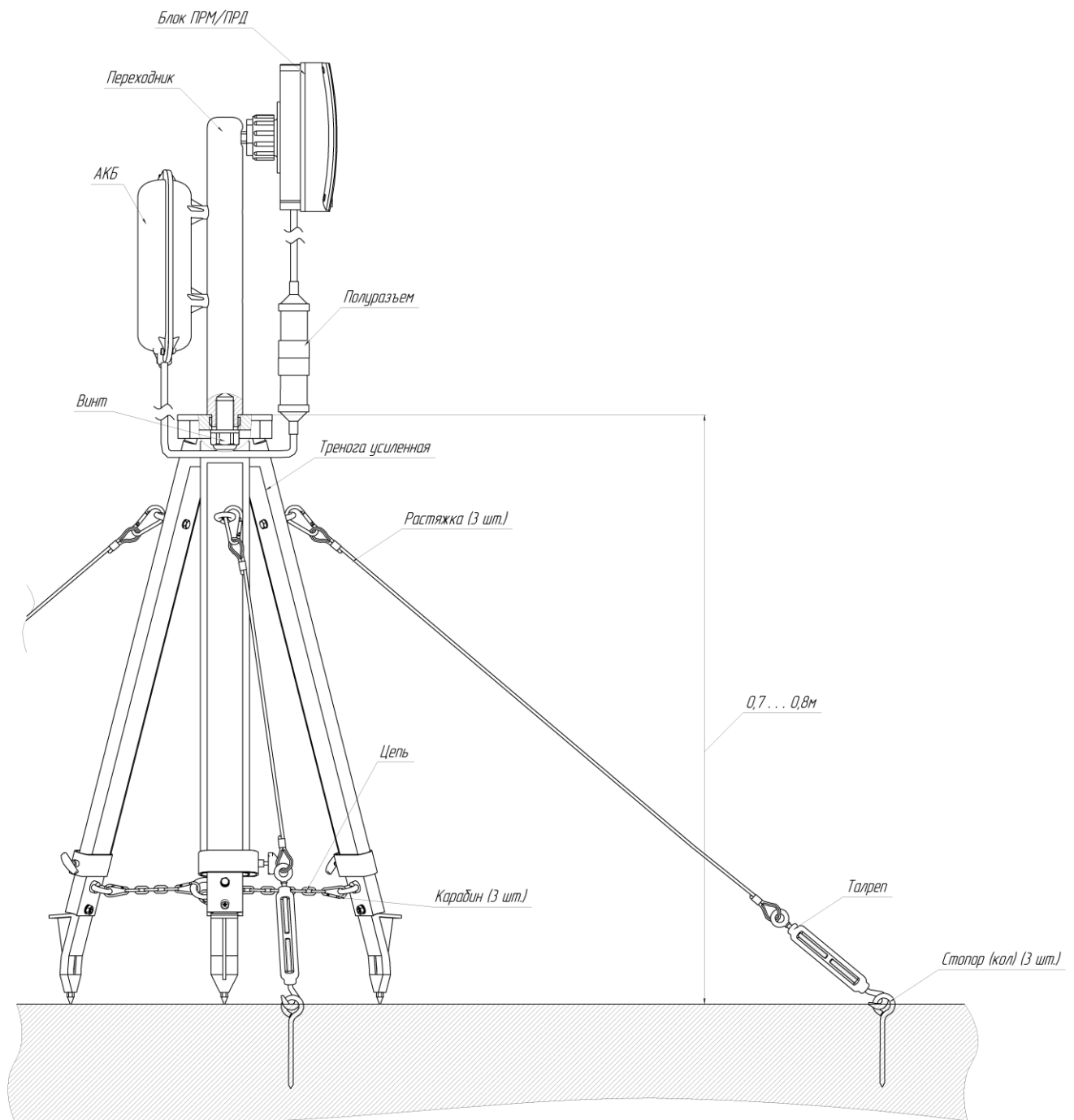
Рисунок 1.11 – Внешний вид блока РЛ, установленного на усиленной треноге, зафиксированной растяжками
