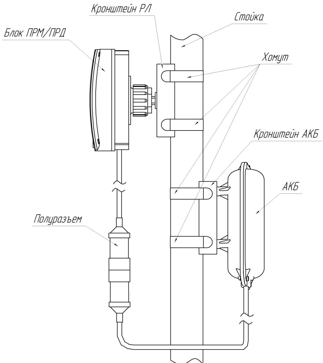
Рисунок 1.10 – Внешний вид блока РЛ, установленного на стационарной стойке
