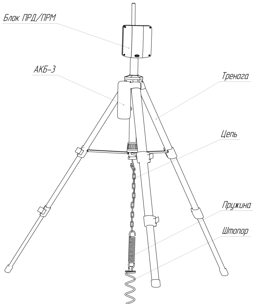
Рисунок 1.6 – Внешний вид ПРМ/ПРД РЛ, установленного на треногу
