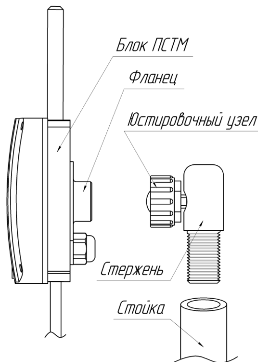
Рисунок 1.16 – Крепление ПСТМ на стойке
