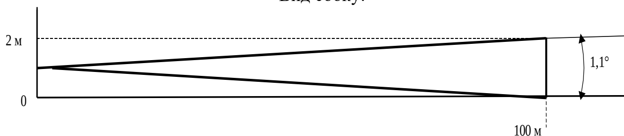
Рисунок 2.4 – Зона обнаружения ИК
