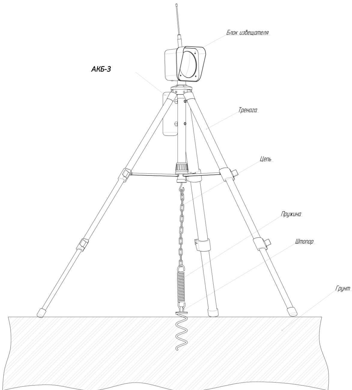
Рисунок 1.12 – Внешний вид извещателя ИК
