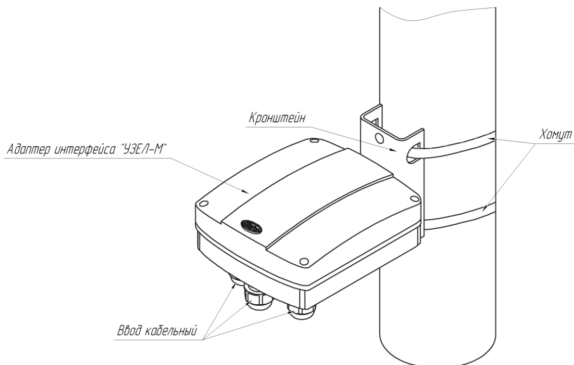
Рисунок 1.2 – Внешний вид изделия, установленного на опоре
