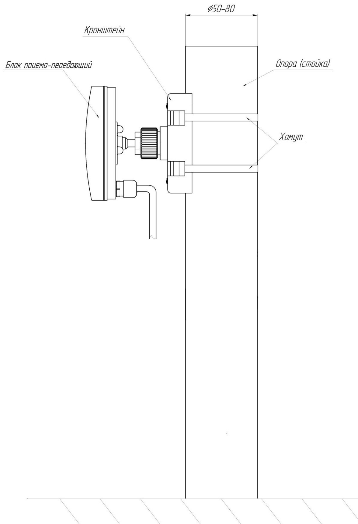
Рисунок 2.1 – Внешний вид блока приема-передающего «АГАТ-СП5У», установленного на опоре
