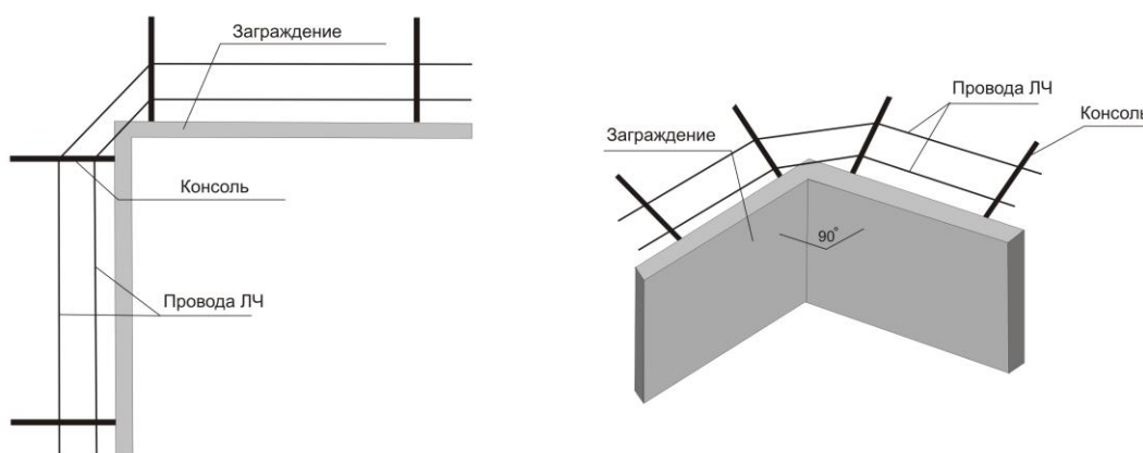
Рисунок Б.2-Блокировка угла с внешней стороны заграждения (вид сверху).
