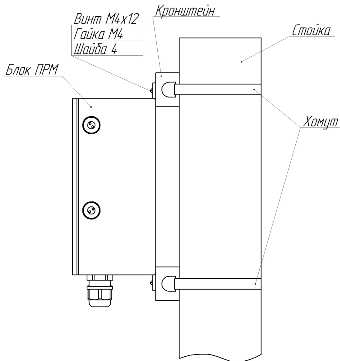
Рисунок 2.1 – Установка блока на опоре (стойке)
