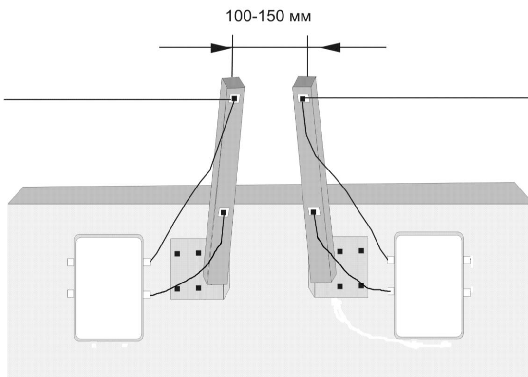
Рисунок Б.5 - Установка консолей на смежных участках
