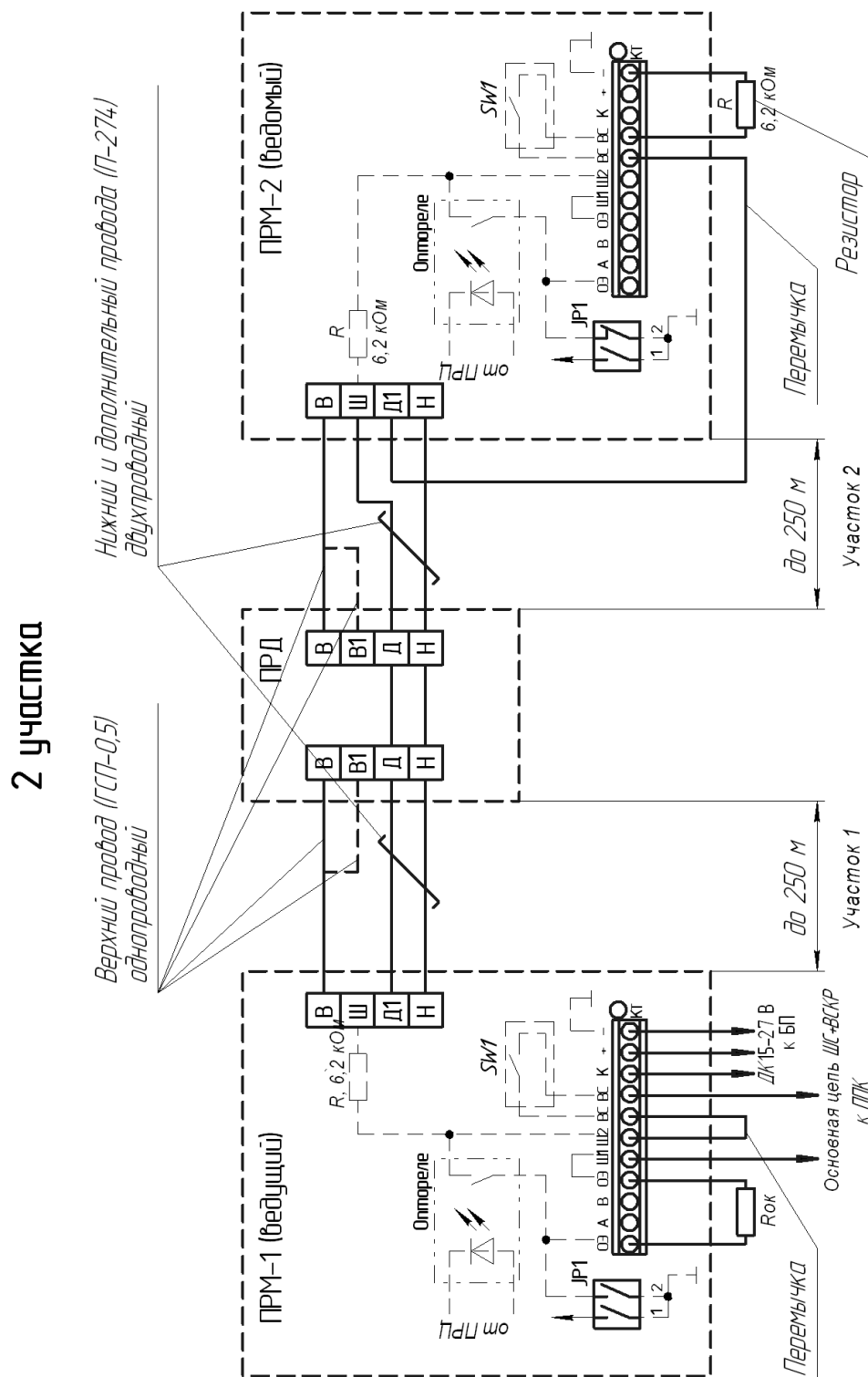
Рисунок В.1 – Схема двухфлангового подключения извещателя
