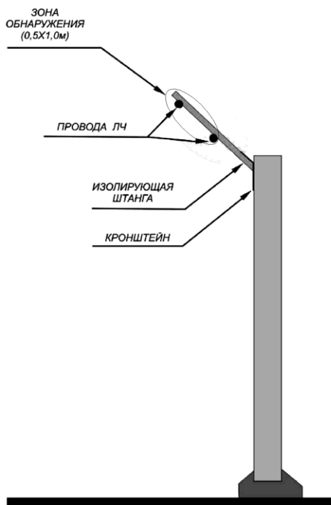
Рисунок А.2 – ЗО при козырьковом варианте применения
