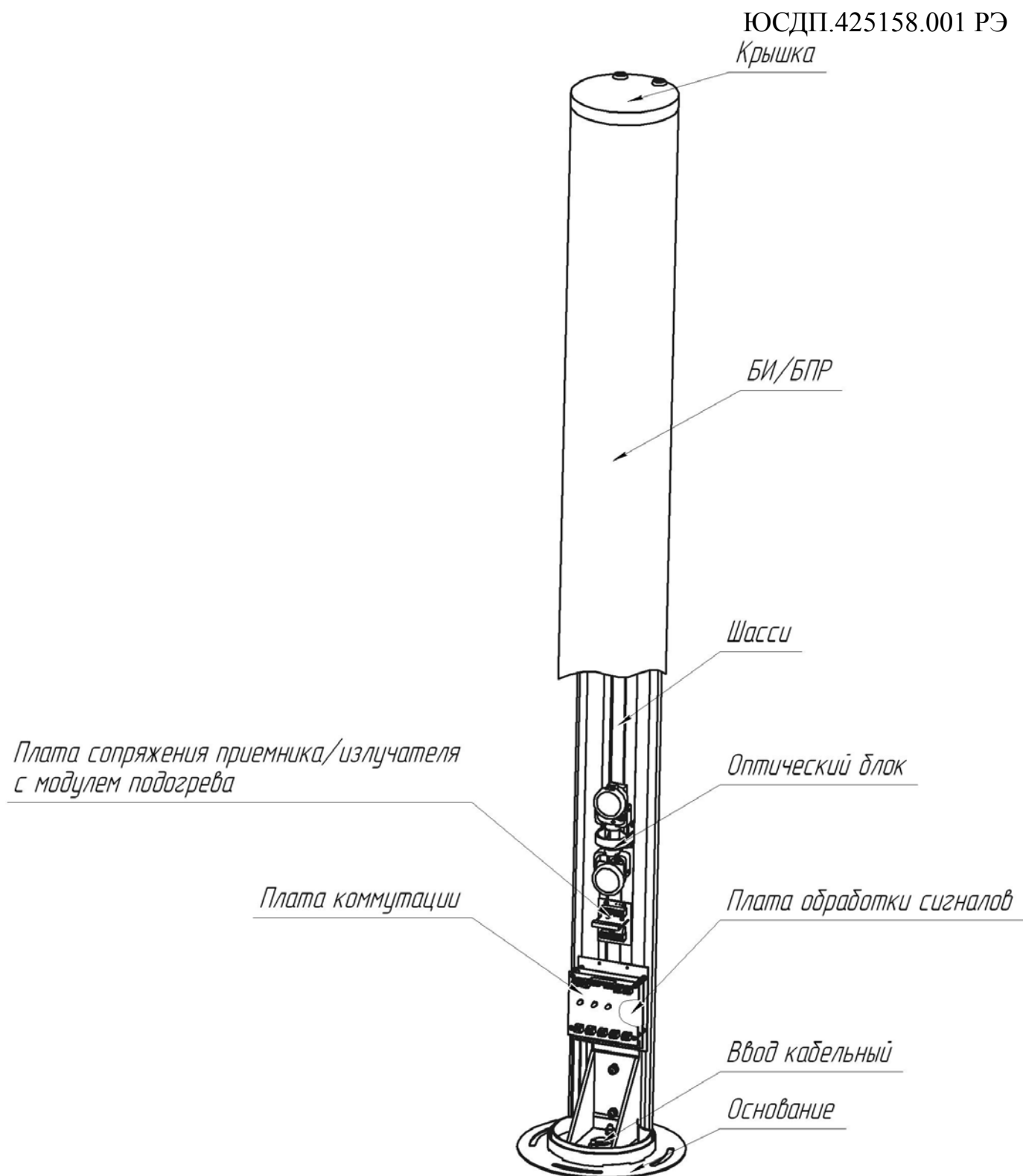
Рисунок 1.3 – Внешний вид БИ/БПР изделия «ПАНТЕРА»
