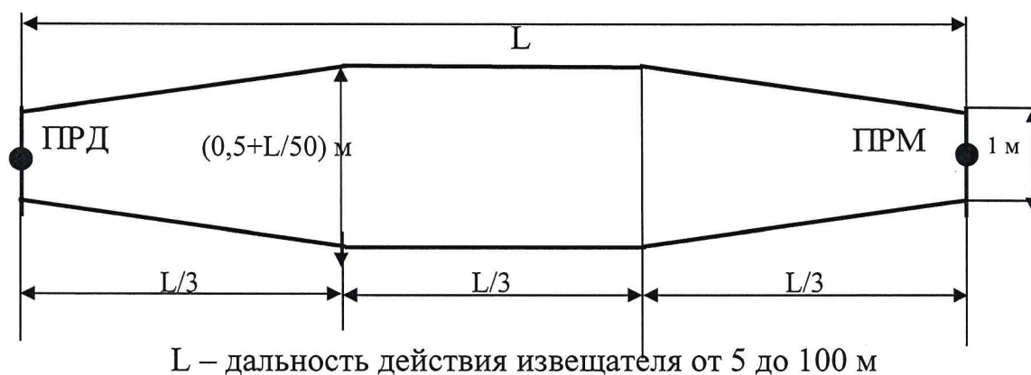
Рисунок 2.1 – Конфигурация и размеры участка для установки извещателя РЛ
