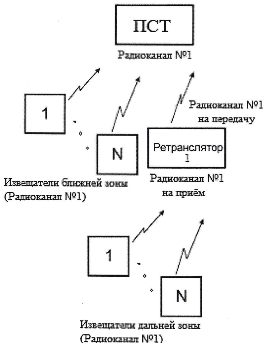
Рисунок 2.7 – Структура комплекса при одноступенчатой ретрансляции
