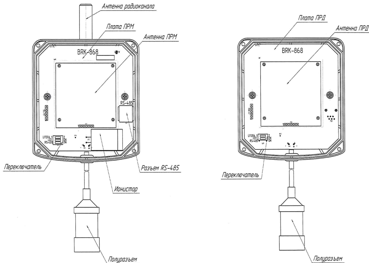
Рисунок 1.8 – Блоки ПРМ и ПРД со снятой крышкой
