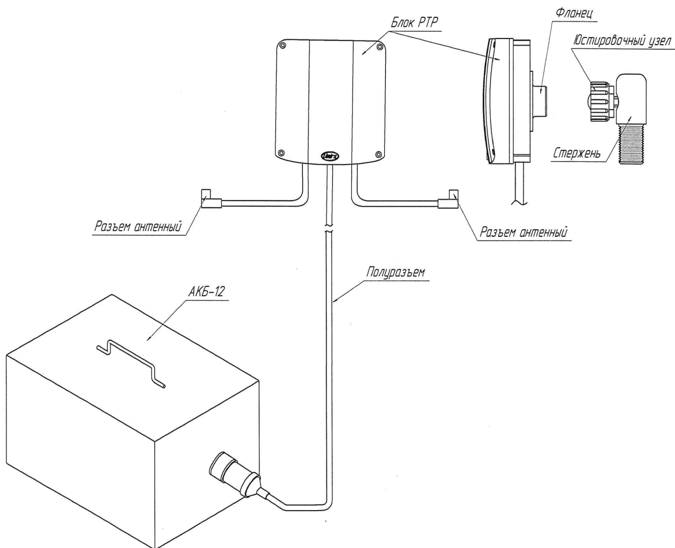
Рисунок 1.19 – Основные элементы РТР
