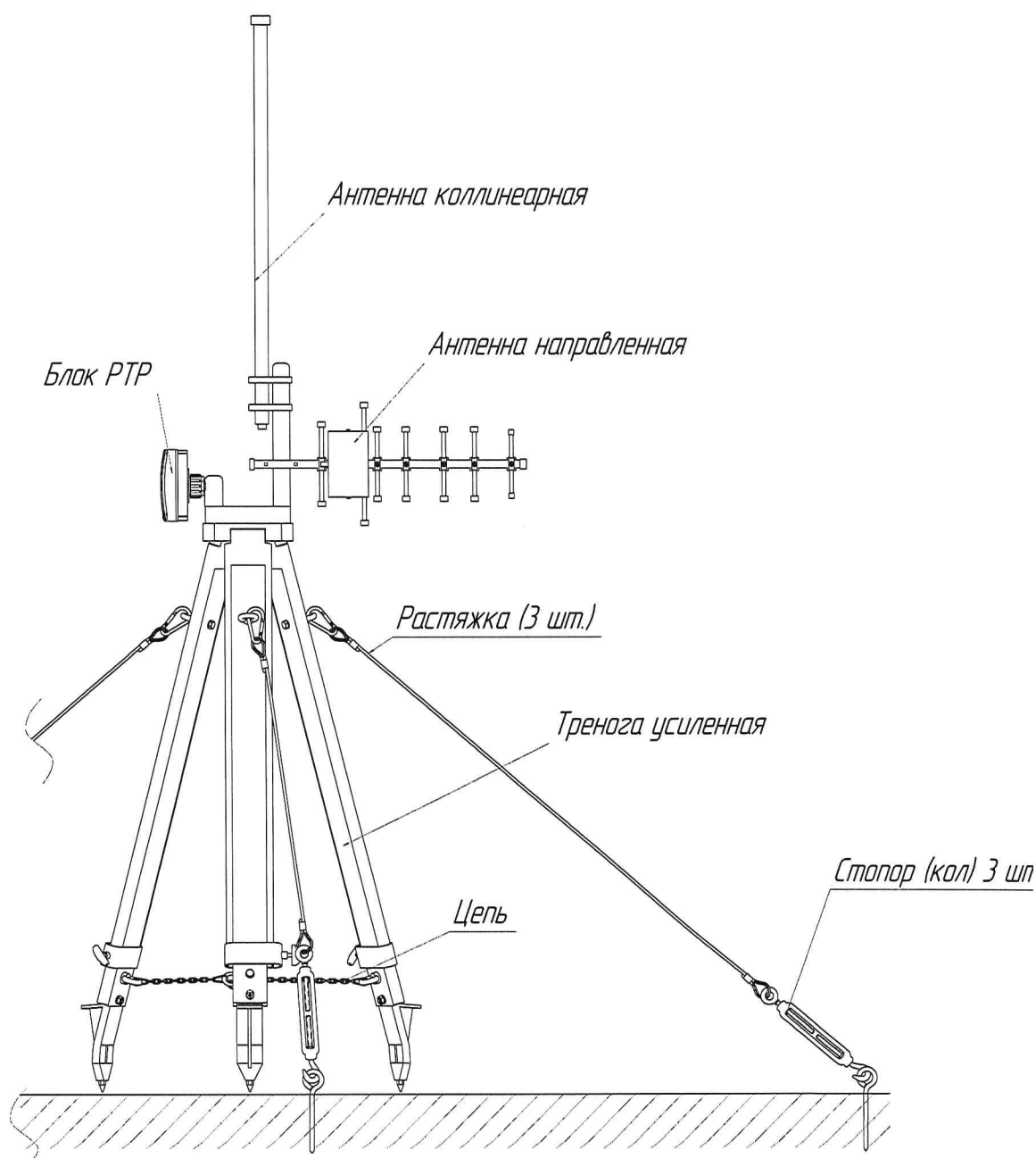
Рисунок 1.18 – Внешний вид РТР, установленного на треноге
