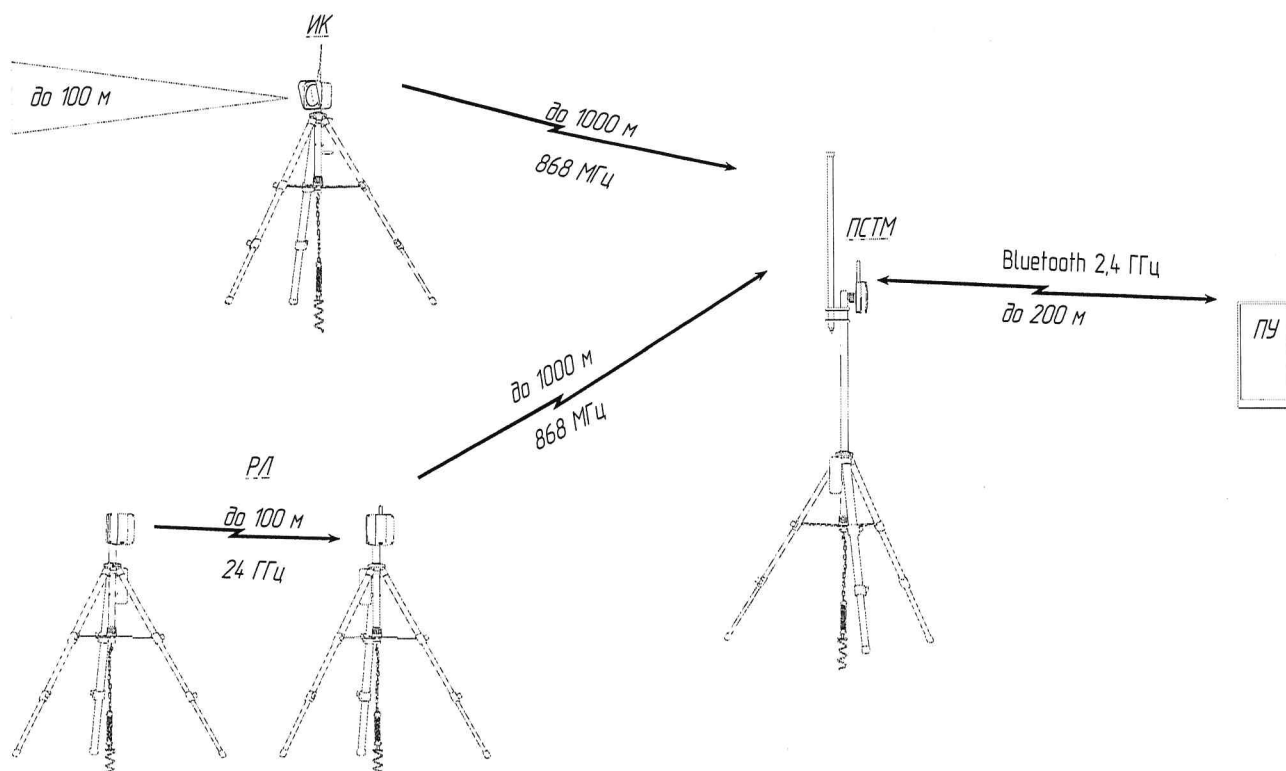
Рисунок 1.4 – Схема взаимодействия составных частей комплекса без RTP (комплект приемника на базе ПСТМ+ПУ)
