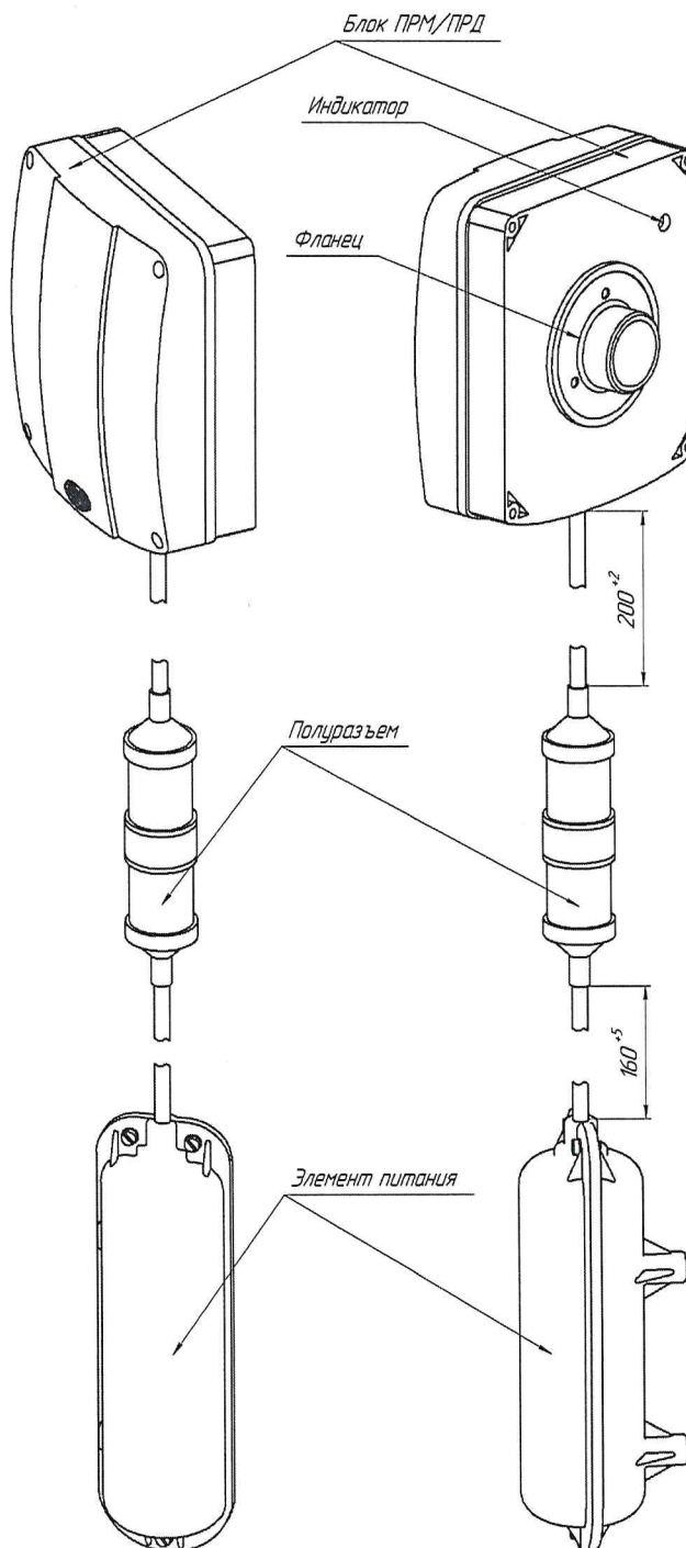
Рисунок 1.7 – Внешний вид ПРМ/ПРД с ЭП
