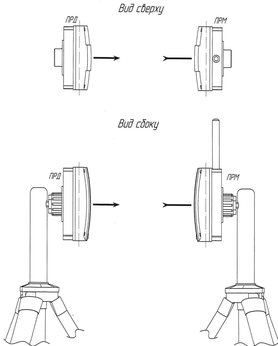
Рисунок 2.3 – Ориентация блоков извещателя РЛ
